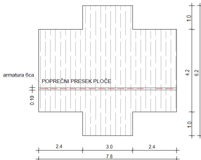
Poprečni presek ploče bazena 7.3x3,75x1,2
